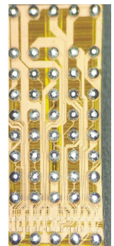
256Mb RPC DRAM DIE & WLCSP
